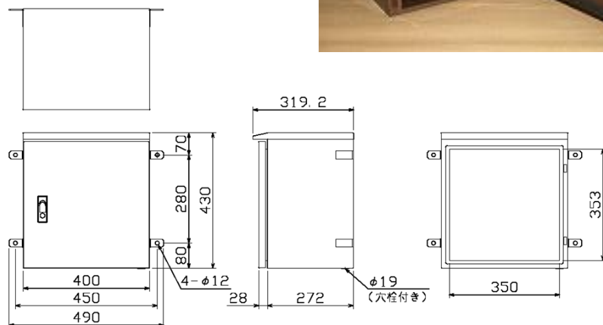
外観寸法図
