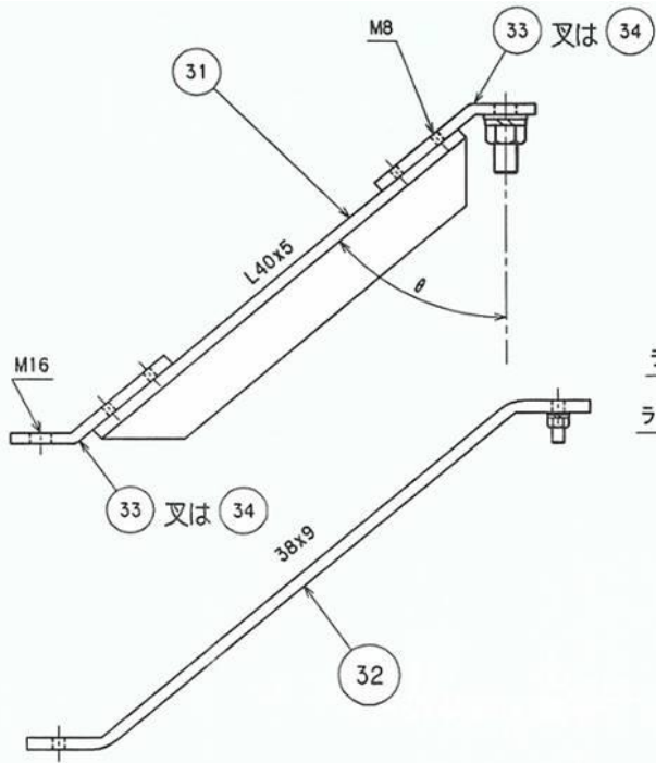
31. 振れ止め金物 材料:山形鋼L40×5
