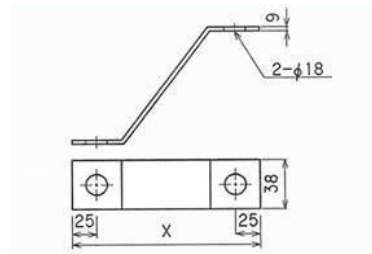
32. 振れ止め金物 材料:平鋼38×9
