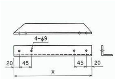
31. 振れ止め金物 材料:山形鋼L40×5
