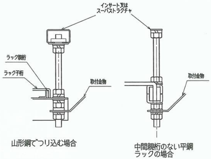
32. 振れ止め金物 材料:平鋼38×9
