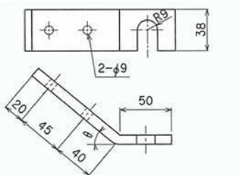
34. 振れ止め金物
