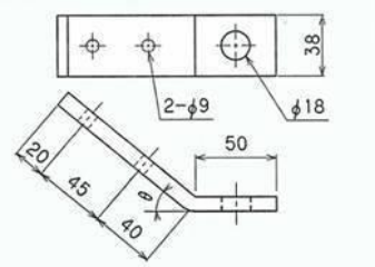
33. 振れ止め金物
